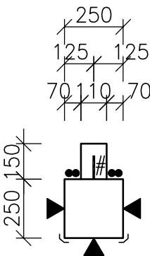
ŘEZ A-A
